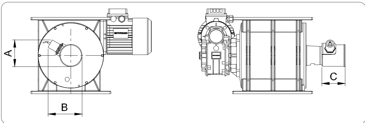
OVERALL DIMENSION - EINBAUMASSE - ENCOMBREMMENT - INGOMBRI
